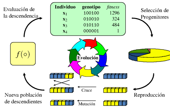
Figura 2.4: Diagrama de flujo del ciclo evolutivo de un algoritmo genético. Tomada de [77].
