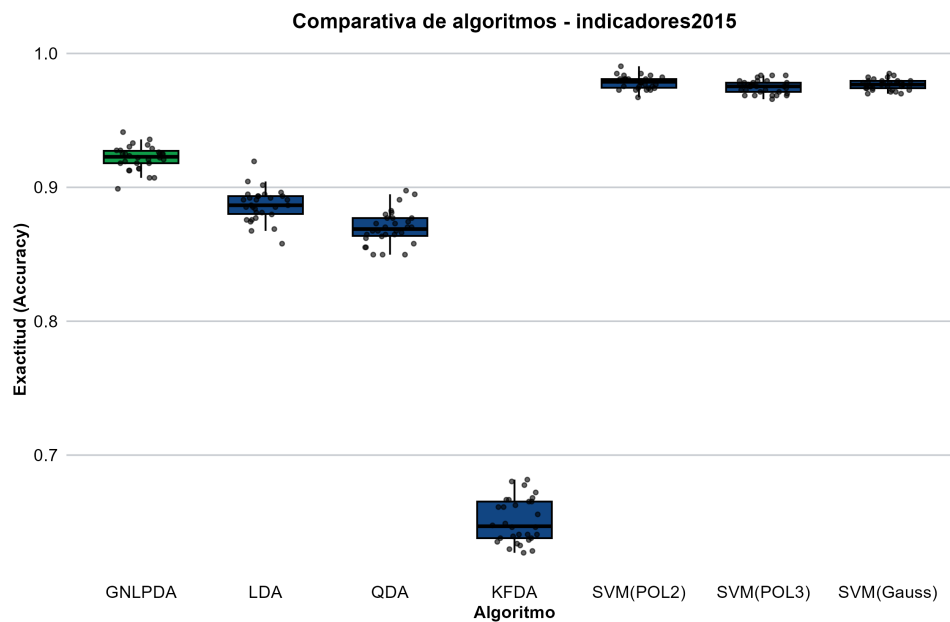
Figura 5.49: Distribución empírica del rendimiento predictivo para el conjunto de datos Indicadores 2015.
