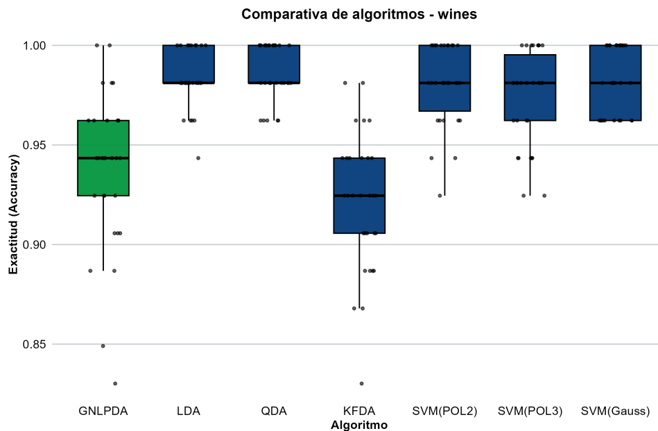
Figura 5.13: Distribución empírica del rendimiento predictivo para el conjunto de datos Wines.
