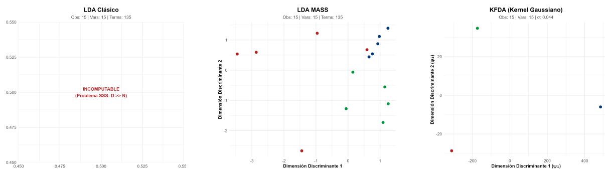
Figura 5.5: Comparativa de los espacios latentes generados por LDA, LDA MASS y KFDA ante el impacto de la alta dimensionalidad (caso 5).
