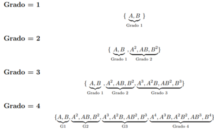
Figura 2.2: Ejemplo de términos generados mediante expansión polinomial para dos variables. Elaboración propia.
