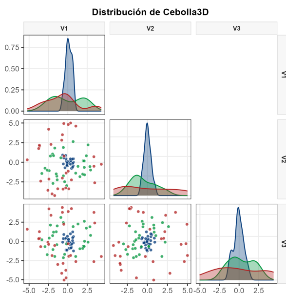
Figura 5.26: Gráficos de dispersión por pares de Cebolla3D.
